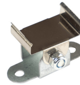
Clip de rotación ECO-X-CLIP-M1 Multi angle clip
